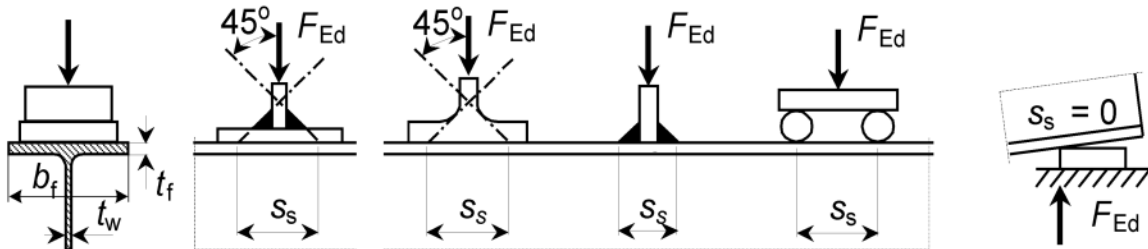
Bild 6.31 — Lasteinleitungslänge
