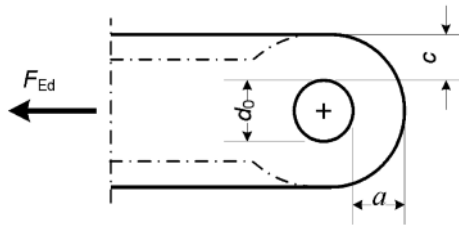
a) Lochdurchmesser und Dicke vorgegeben
