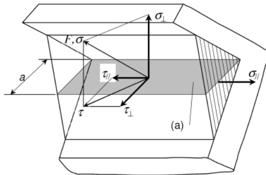
(a) Nahtquerschnitt
