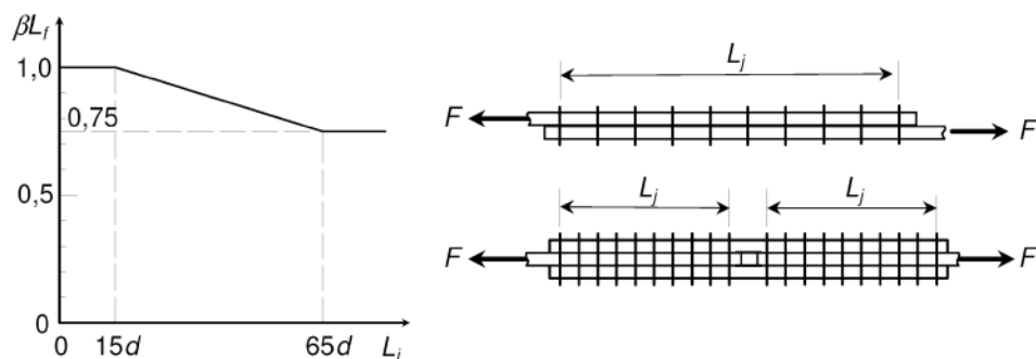
Bild 8.10 — Lange Anschlüsse
