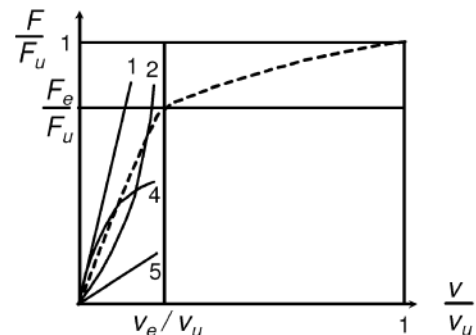
Bild L.3 — Wichtige Verbindungstypen
