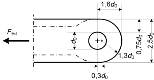
b) Geometrie vorgegeben
