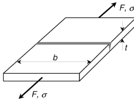
Bild 8.14 — Stumpfnah mit Normalspannungen
