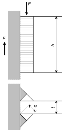
Bild 8.20 — Doppelkehlnahtanschluss mit Beanspruchung parallel zur Schweißnahtachse
