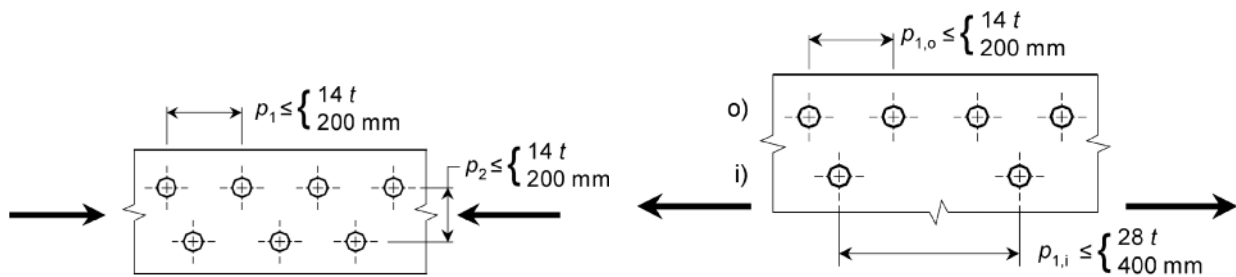
Bild 8.1 — Bezeichnungen der Abstände zwischen Verbindungsmitteln
