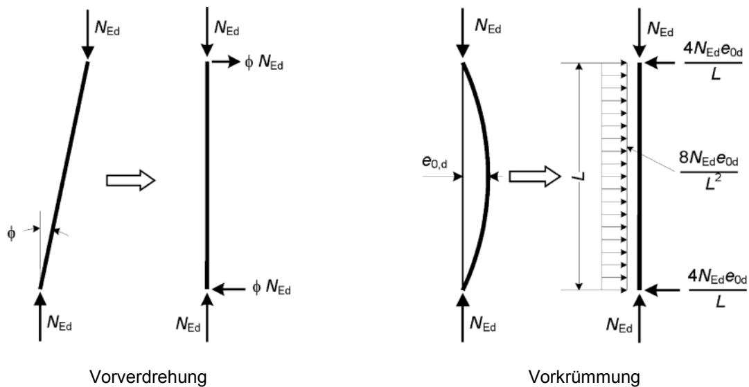
Bild 5.3 — Ersatz der Vorverformungen durch äquivalente horizontale Ersatzlasten
