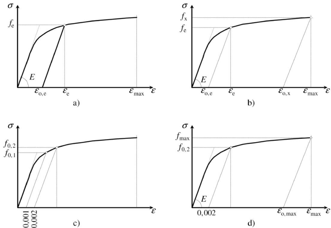
Bild E.4 — Kontinuierliche Modelle der Form \epsilon = \epsilon(\sigma)
