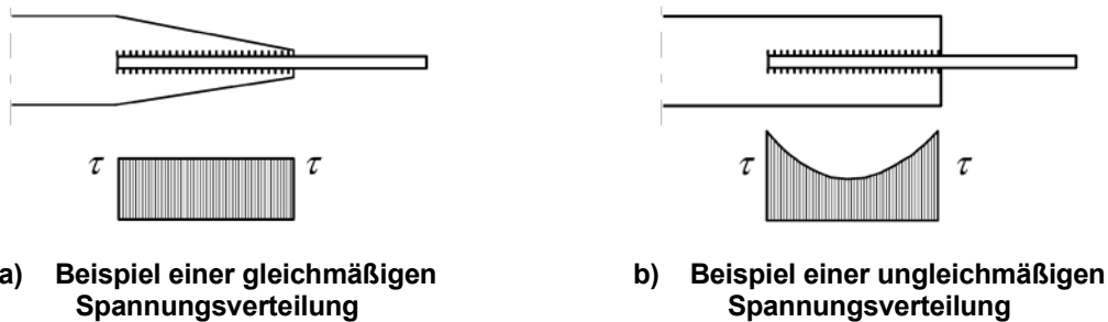
Bild 8.16 — Spannungsverteilungen in Verbindungen mit Kehlnähten A1
