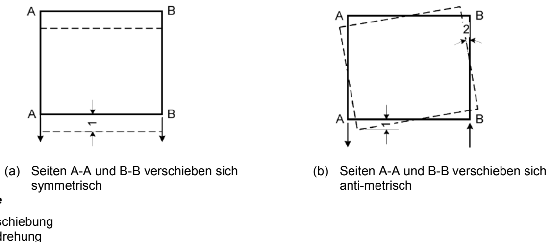
Bild 5.4 — Verschiebungsmöglichkeiten und Einflüsse aus Torsion (Draufsicht)
