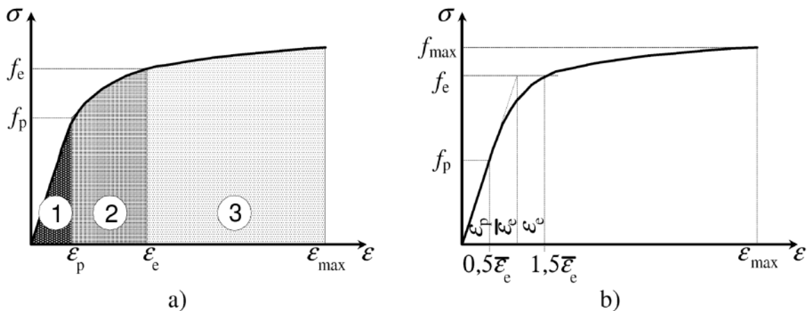
Bild E.3 — Kontinuierliche Modelle der Form \sigma = \sigma(\varepsilon)
