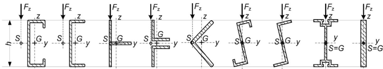
Bild I.2 — Träger mit konstantem Querschnitt, der zur starken Achse symmetrisch, zentralsymmetrisch oder doppeltsymmetrisch ist
