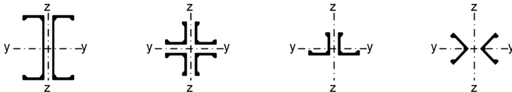
Bild 6.20 — Mehrteilige Bauteile mit geringer Spreizung
