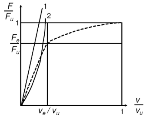
Bild L.3 — Wichtige Verbindungstypen
