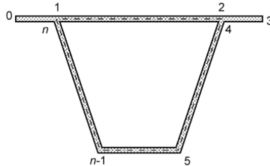
Bild J.5 — Querschnitt mit geschlossener Zelle
