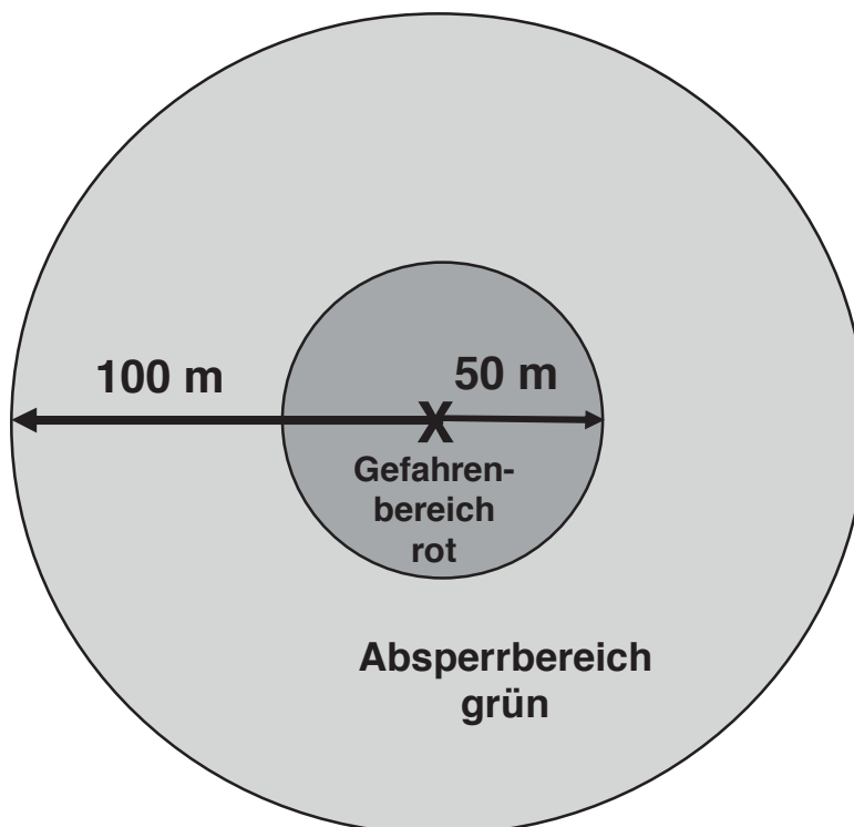
Schematische Darstellung von Gefahren- und Absperrbereich
